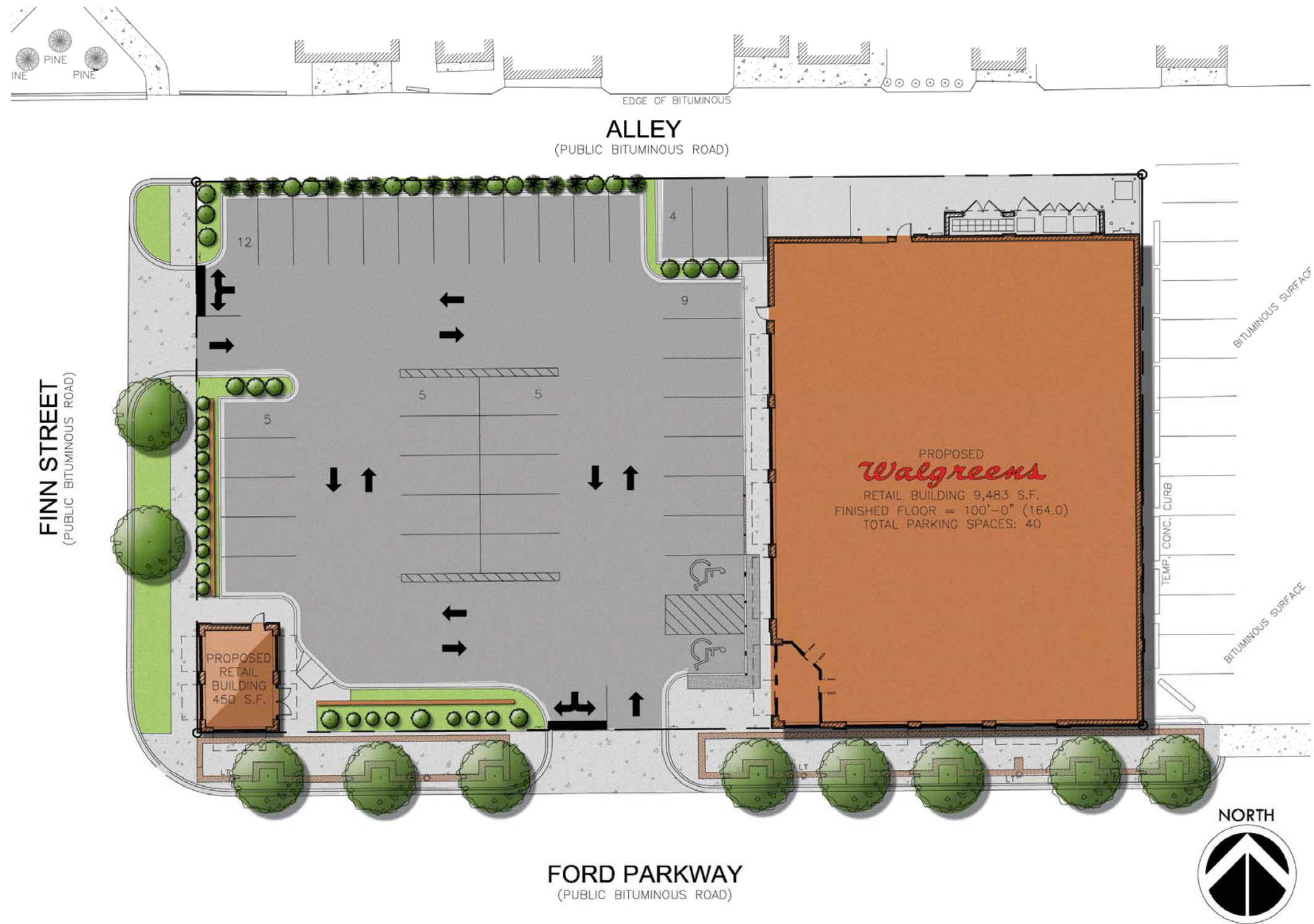
COLOR SITE PLAN
